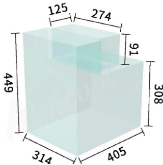
Medidas interiores
